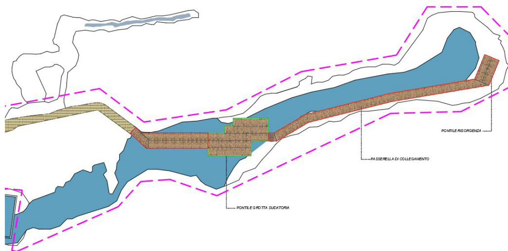
Fig. 6 - Planimetria generale della grotta sudatoria con indicazione del perimetro della grotta, il posizionamento e l'estensione della passerella e del corso d'acqua termale.
