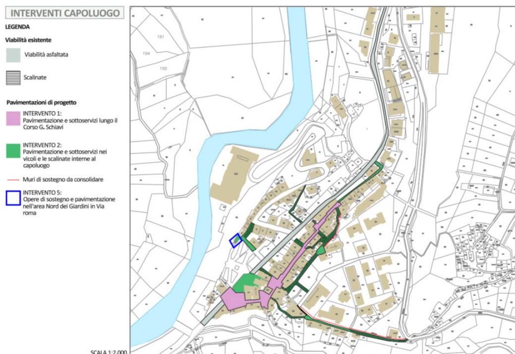
Fig. 4 - Planimetria con individuazione interventi oggetto di analisi e progettazione nel capoluogo di Acquisanta Terme.
