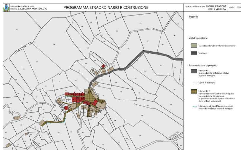
Fig. 3 - Planimetria degli interventi di pavimentazione e realizzazione delle opere di sostegno interne alla frazione e lungo la viabilità di accesso, estratta dal PSR, non cogente rispetto alle estensioni programmate.
