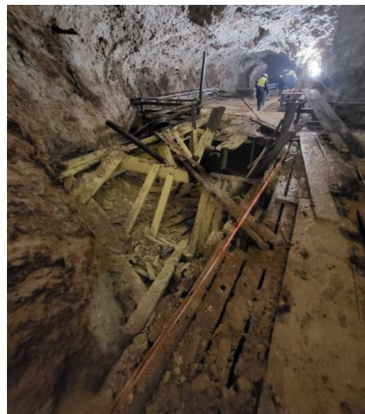
Fig. 8 - Foto dello stato di fatto della passerella.
